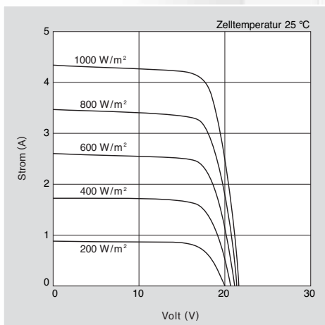
Strom-Spannungs-Kennlinie des Moduls KC70 bei verschiedener Einstrahlung.
