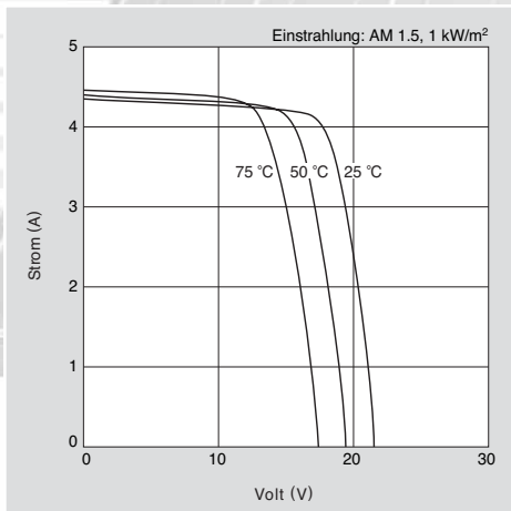
Strom-Spannungs-Kennlinie des Moduls KC70 bei verschiedenen Zelltemperaturen.
